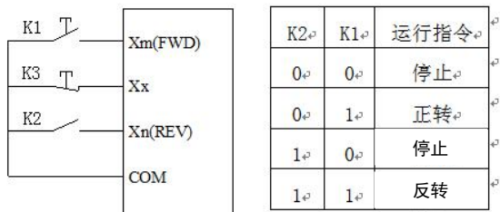
图 F4-5 三线式控制模式 2 示意图
