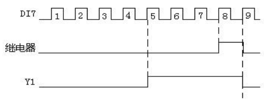
图 FB-2 计数器复位设定和计数器检测设定示意图
