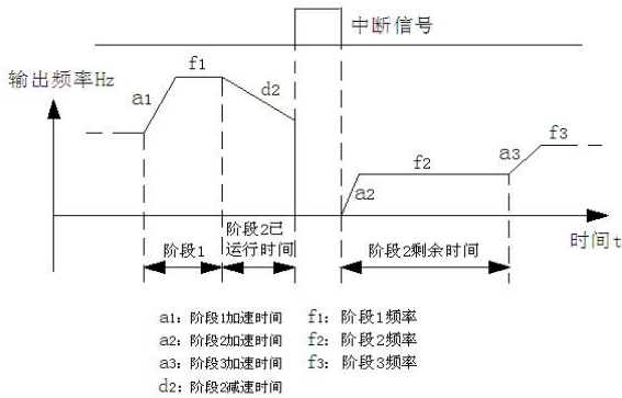
图 FC-5 PLC 起动方式 2
