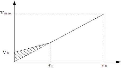
Vb-手动转矩提升量，fz-转矩提升截止频率 图 F3-3 转矩提升示意图
