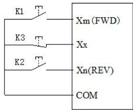
图 F4-4 三线式控制模式 1 示意图
