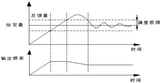
图 FA-3 偏差极限示意图
