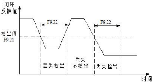
图 F9-4 闭环反馈丢失检出时序图
