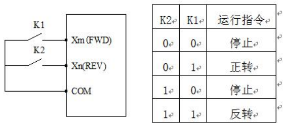
图 F4-3 二线式控制模式 2 示意图
