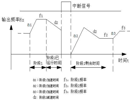
图 FC-4 PLC 起动方式 1
