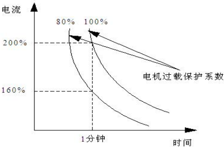
图 F9-1 电机过载保护曲线
