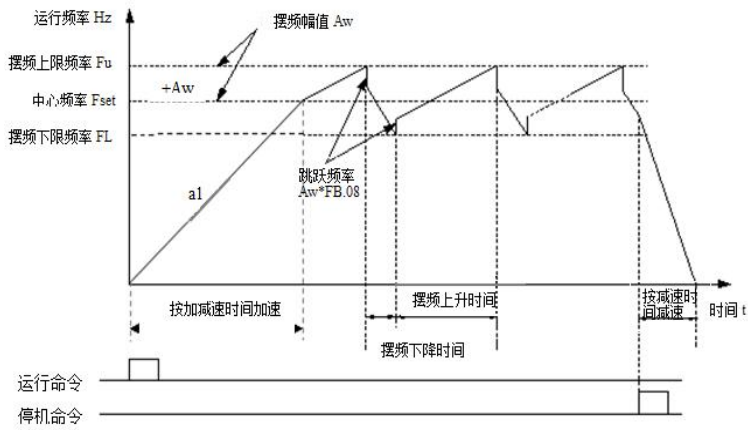
图 FB-1 摆频示意图
