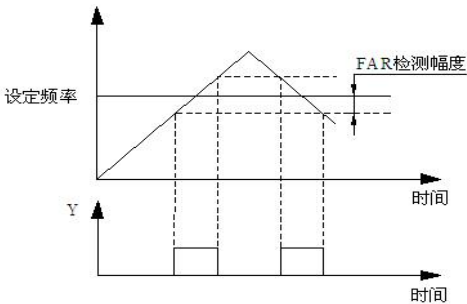
图 F8-4 频率到达示意图
