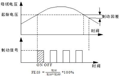
图 FE-1 能耗制动示意图
