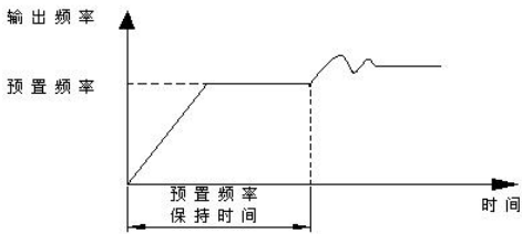
图 FA-4 闭环预置频率运行示意图
