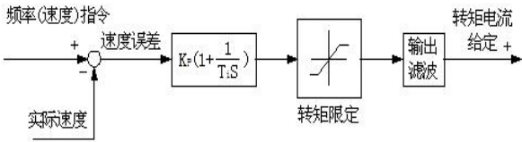
图 F2-1 速度调节器简化图
