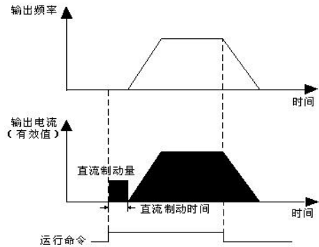
图 F6-2 起动直流制动示意图
