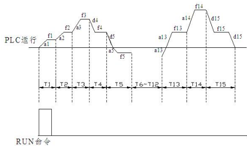
图 FC-1 PLC 单循环后停机示意图
