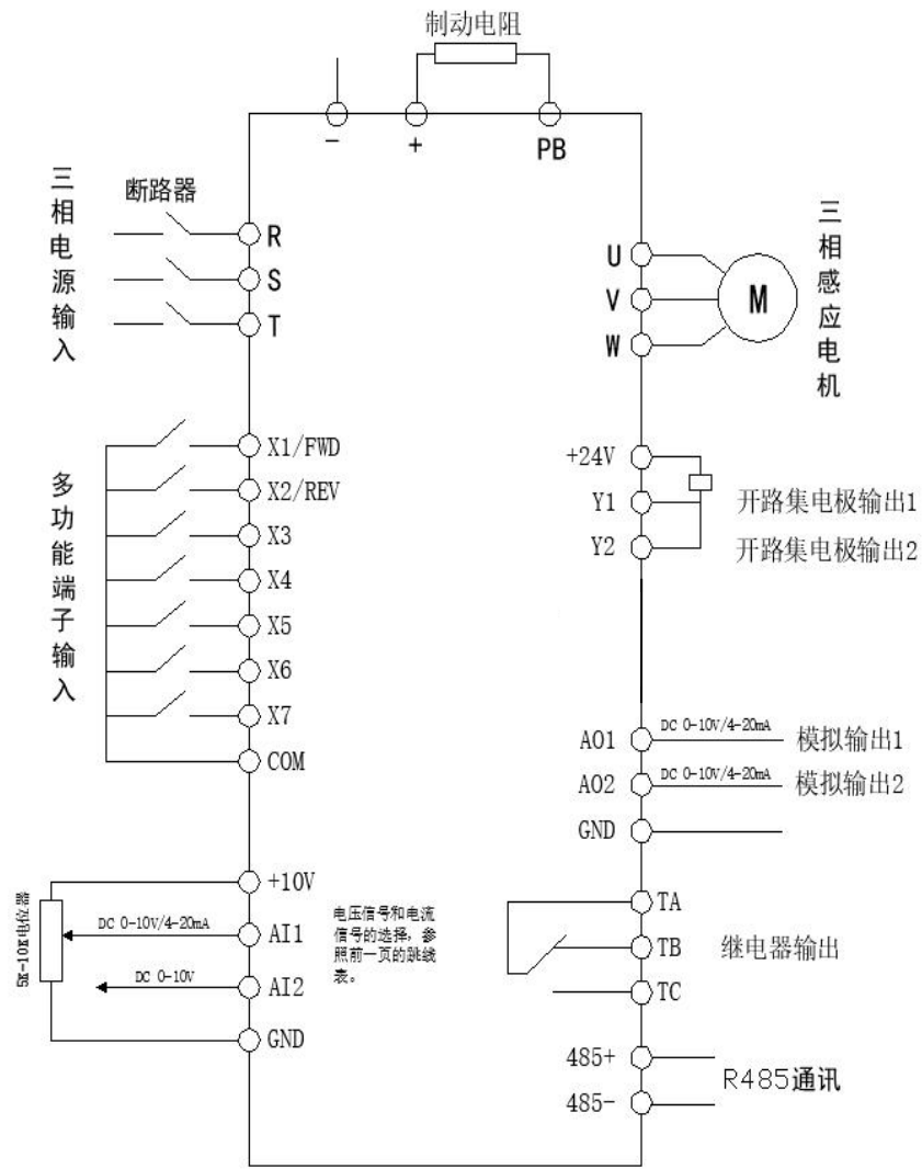
基本运行配线图
