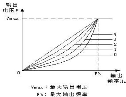
图 F3-1 V/F 曲线示意图
