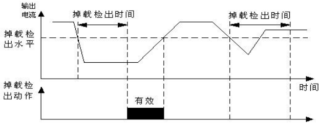
图 F9-3 掉载检出示意图
