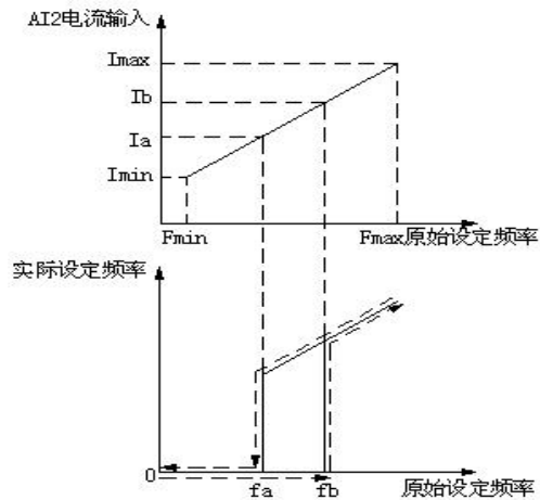
fb：零频运行阈值 fa：fb - 零频回差
