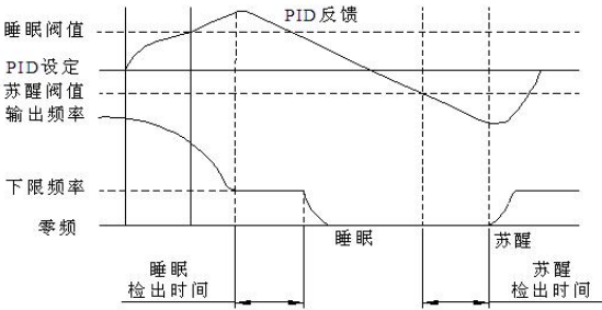
图 FA-5 第一种睡眠模式示意图
