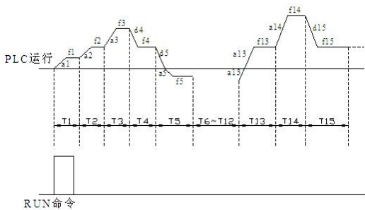
图 FC-3 PLC 连续循环示意图
