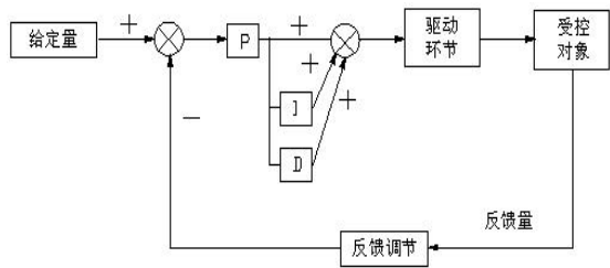
图 FA-2 PID 调节示意图
