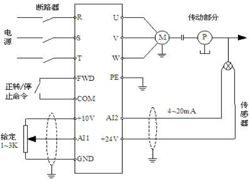
图 FA-1 模拟反馈控制系统示意图
