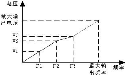
图 F3-4 用户设定 V/F 曲线示意图
