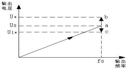
图 F3-5 电压控制模式 0
