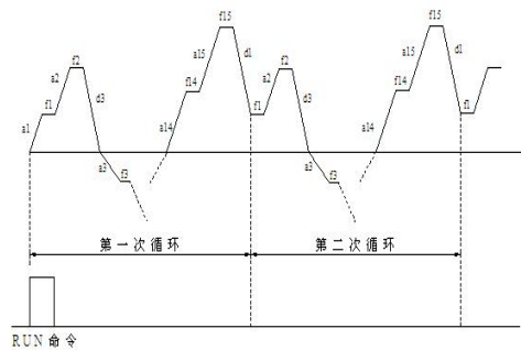
图 FC-2 PLC 单循环后保持示意图
