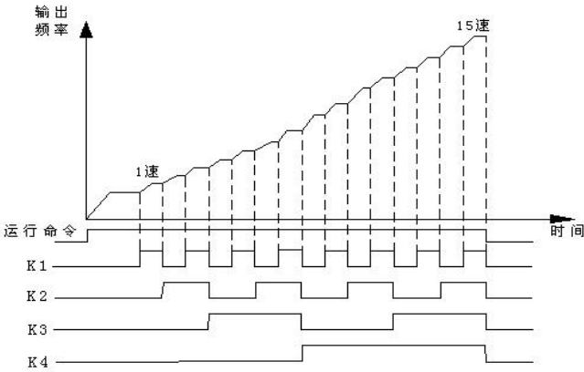
图 F4-1 多段速运行示意图
