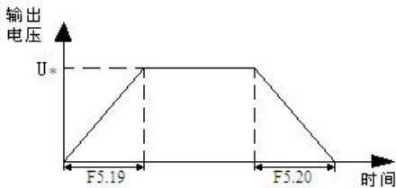
图 F3-6 电压控制模式 1
