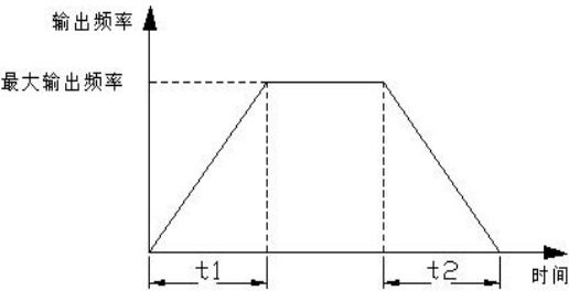
图 F0-2 加速时间和减速时间示意图
