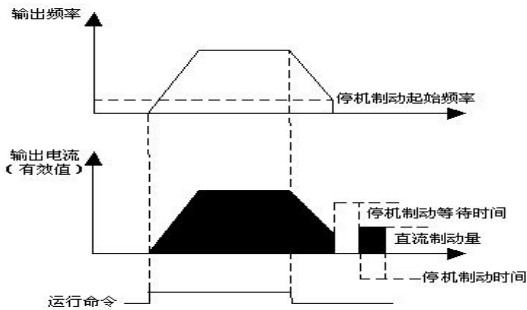
图 F6-4 停机直流制动示意图
