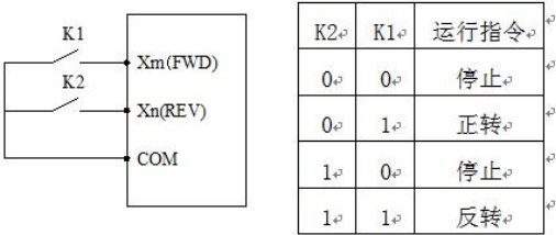
图 F4-2 二线式控制模式 1 示意图
