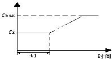
图 F6-1 启动频率示意图
