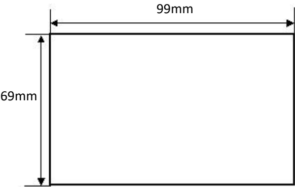
外引键盘安装尺寸
