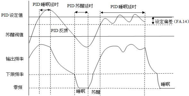
图 FA-6 第二种睡眠模式示意图
