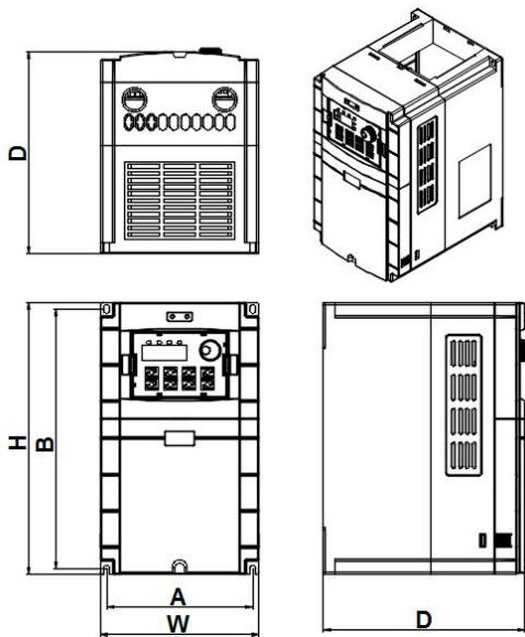
图 D-1 变频器 0.75KW~500KW 尺寸
